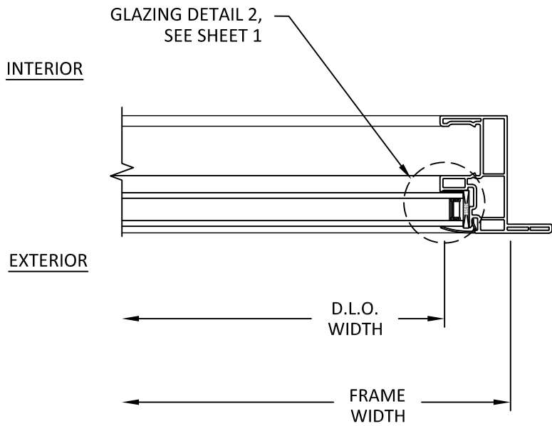
E 4 HORIZONTAL SECTION V152 FRAME - FX JAMB
